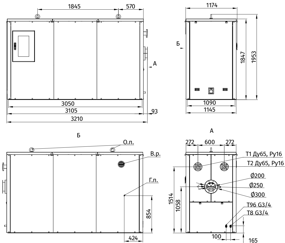
Рисунок 1 - Габаритные и присоединительные размеры
