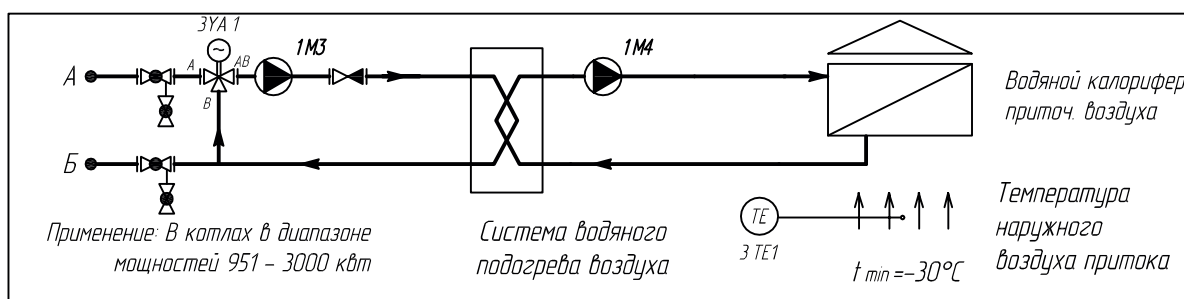
Рисунок 2 - Функционально-структурная схема. Структура КИПиА котла (продолжение)
