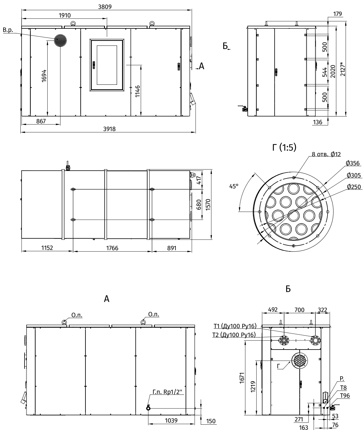
Рисунок 1. Габаритные и присоединительные размеры
