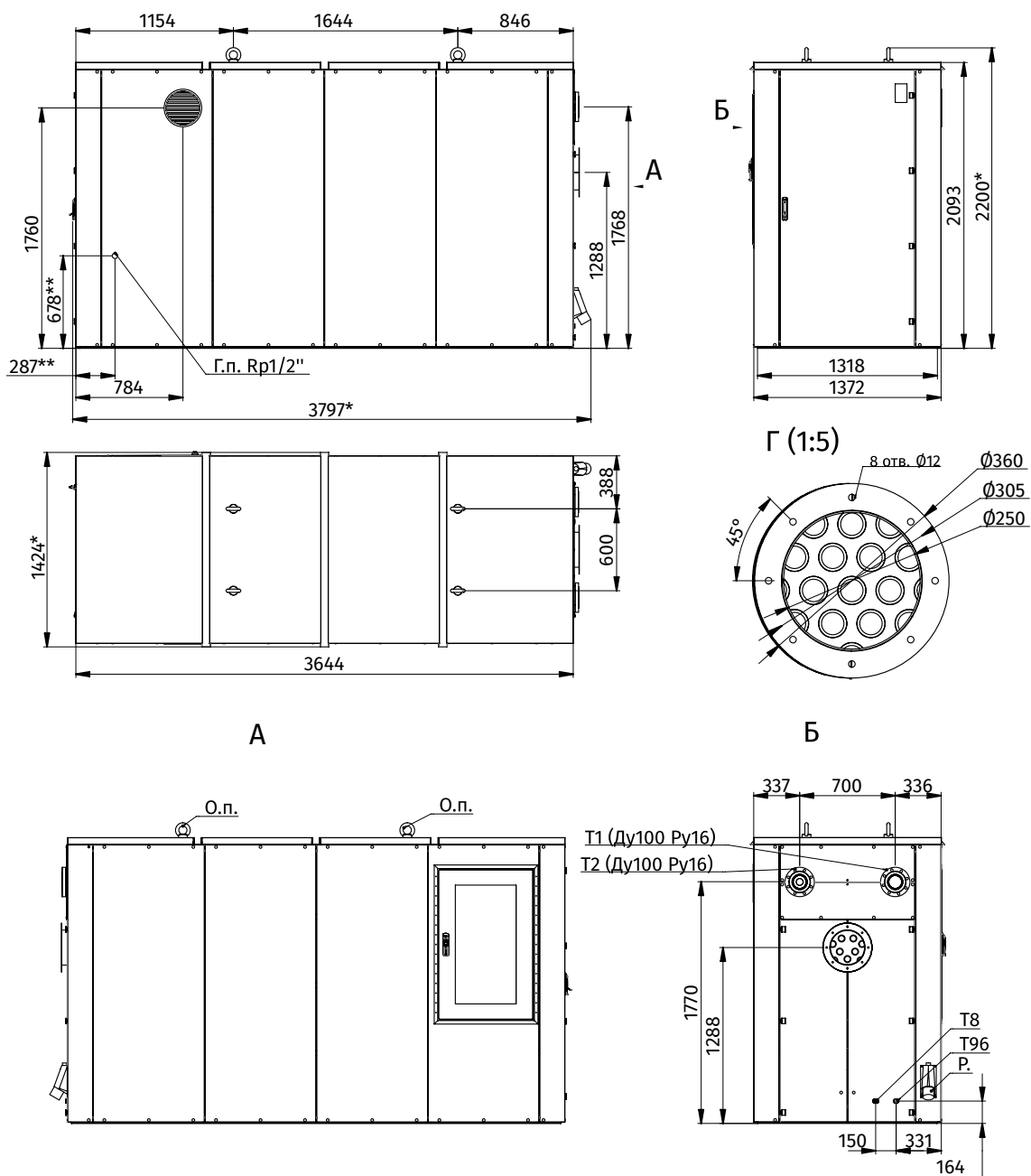
Рисунок 1. Габаритные и присоединительные размеры
